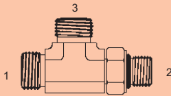
Y-OFS-6804-F-NWO - Tee
