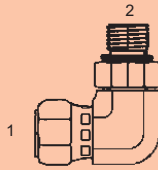
Y-OFS-6809-F-NWO - 90°
