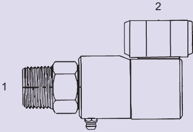
SLS-6573-4K - 90° 4000 PSI (1) Male Pipe - Stem (2) Fem. 37° Swivel - Barrel
