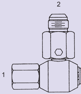
SLS-DP-2581 - 90°
